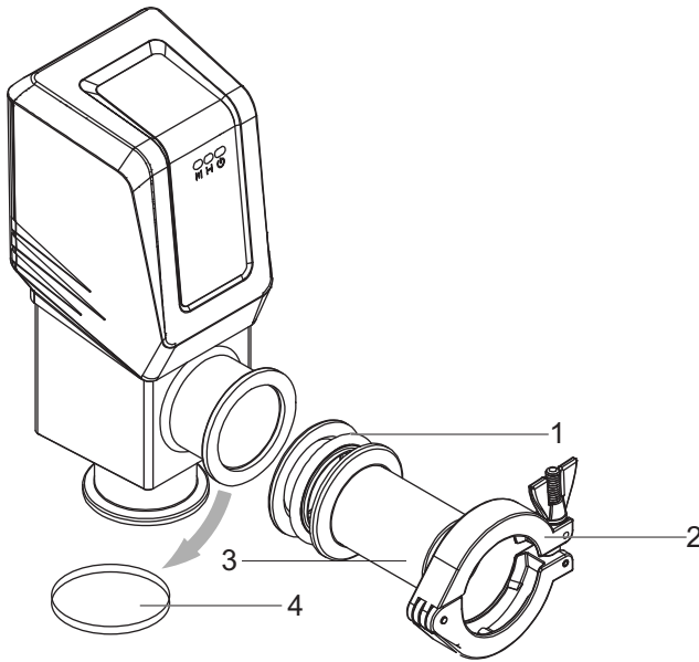
图片 2： 真空连接
