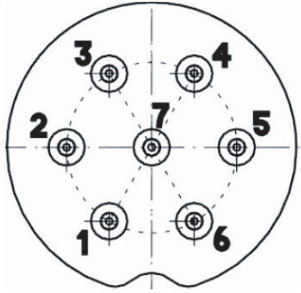
图片 3: 连接器针脚使用
