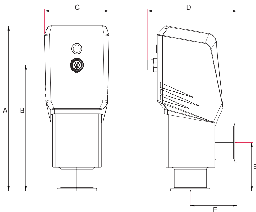
图片 4: E 系列电动角阀尺寸
